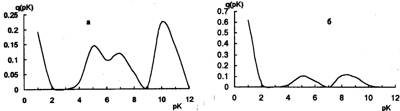
Рис. 4. Типичные рК-спектры гумусовых кислот: а – торфяные ГК; б – речные ГК
