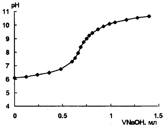
Рис. 1. Типичная кривая потенциометрического титрования выделяющейся уксусной кислоты при определении карбоксильной кислотности ГК Са-ацетатным методом
